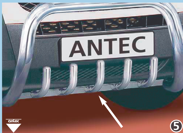
EU-under-ride protection 42mm front (fitting with EU-pedestrian protection guards only) EU-alleajoeste 42mm vorne (nur montierbar mit EU-Personenschutzbügel) Stainless steel / jaloteräs
